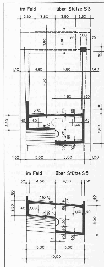
Bild 3. Charakteristische Querschnitte
