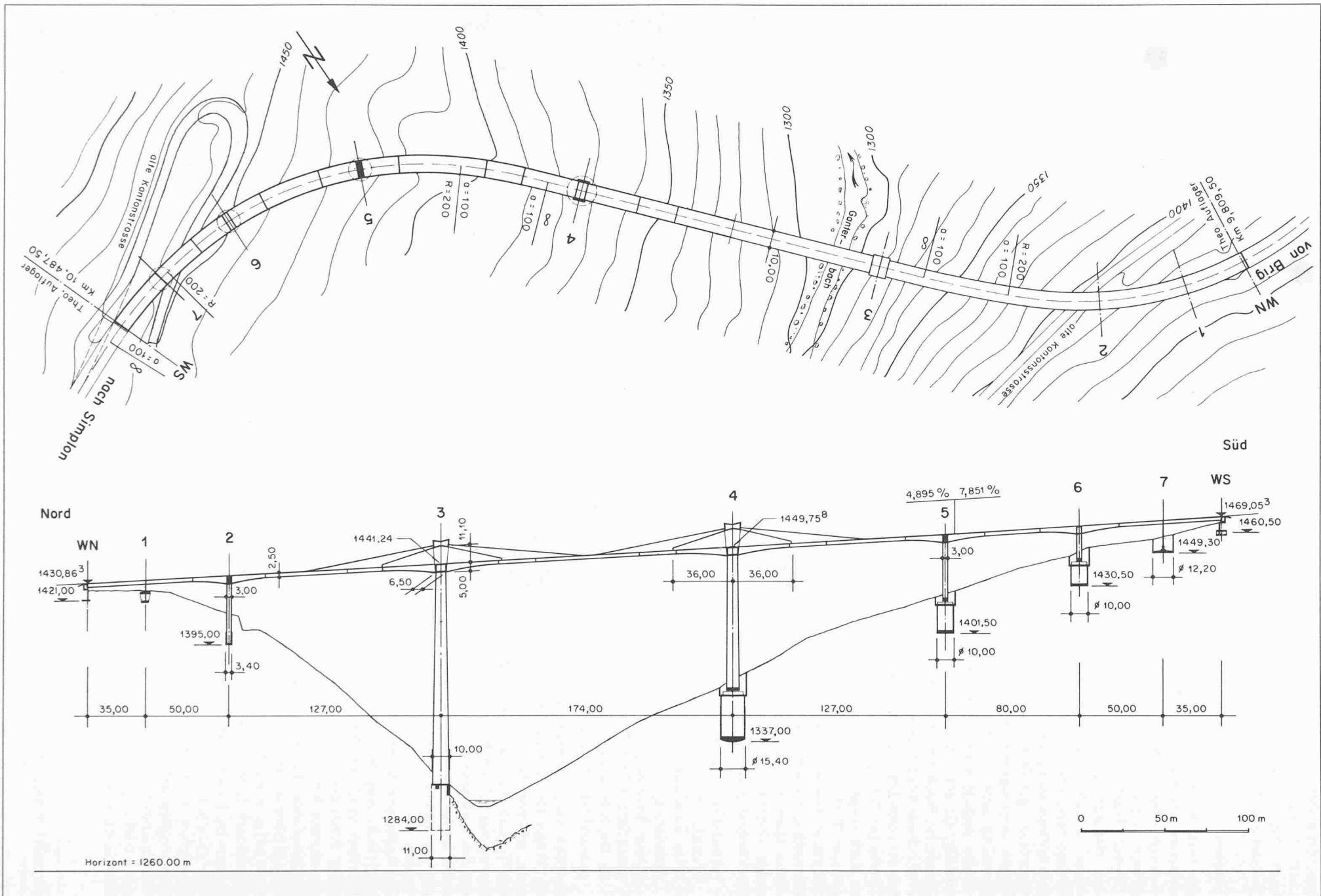
Bild 1. Übersichtsplan
