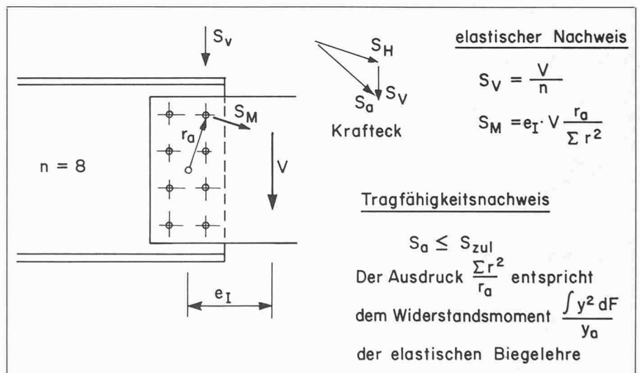
Bild 9. 4. Versuch, geschraubte Stegstöße, elastischer Nachweis
