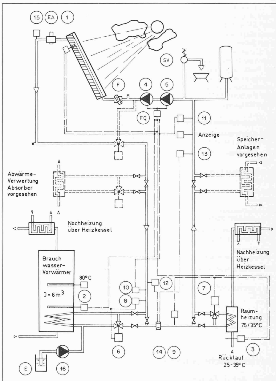
Schema der Sonnen-Mitheizungsanlage, 1. Ausbaustufe
