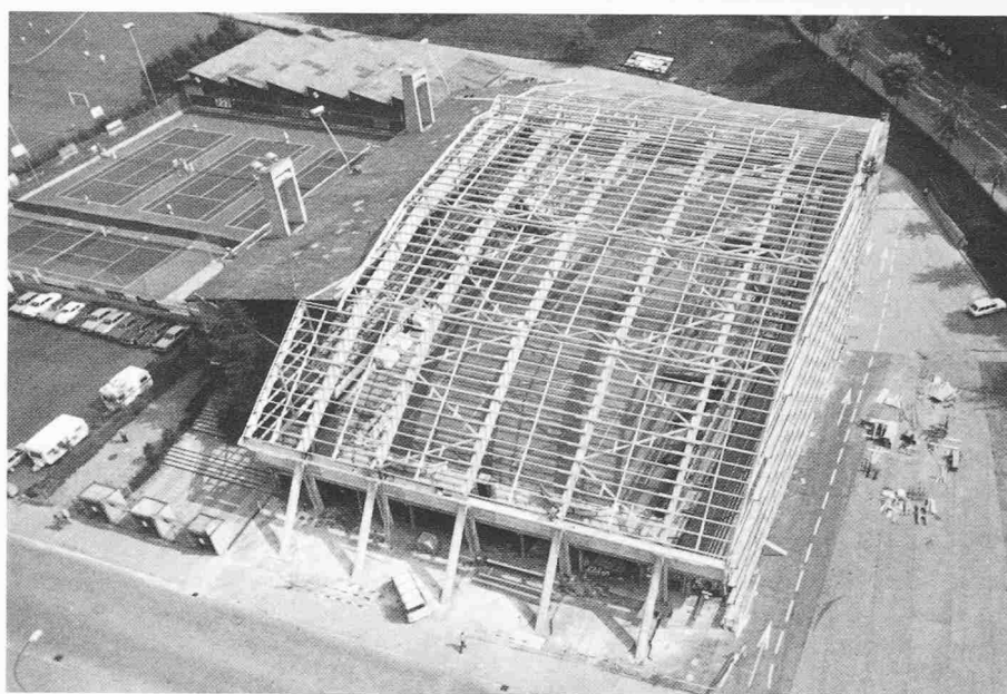
Das Holztragwerk der Eishalle Luzern. Flugaufnahme: Walker/Bahnholzer, Luzern)
