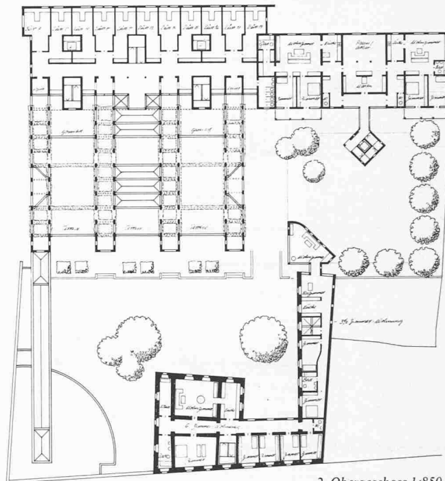
2. Obergeschoss 1:850
