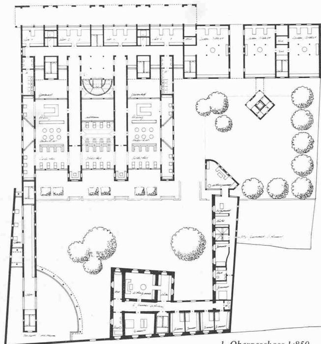
1. Obergeschoss 1:850
