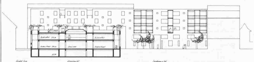
Schnitt/Ansicht Rosshofgasse-Platz 1:850
