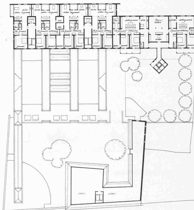
3. Obergeschoss 1:850
