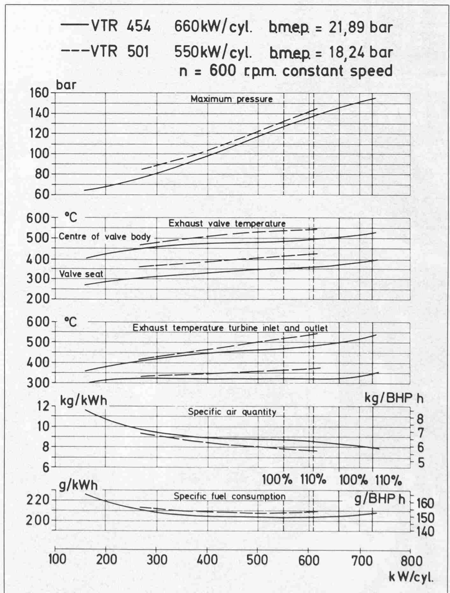
Bild 3. Verbesserung des Betriebsverhaltens eines Sulzer-Dieselmotors 8 ZL 40/48 (aus MTZ, Heft Nov. 11, 1979, Seite 519)
