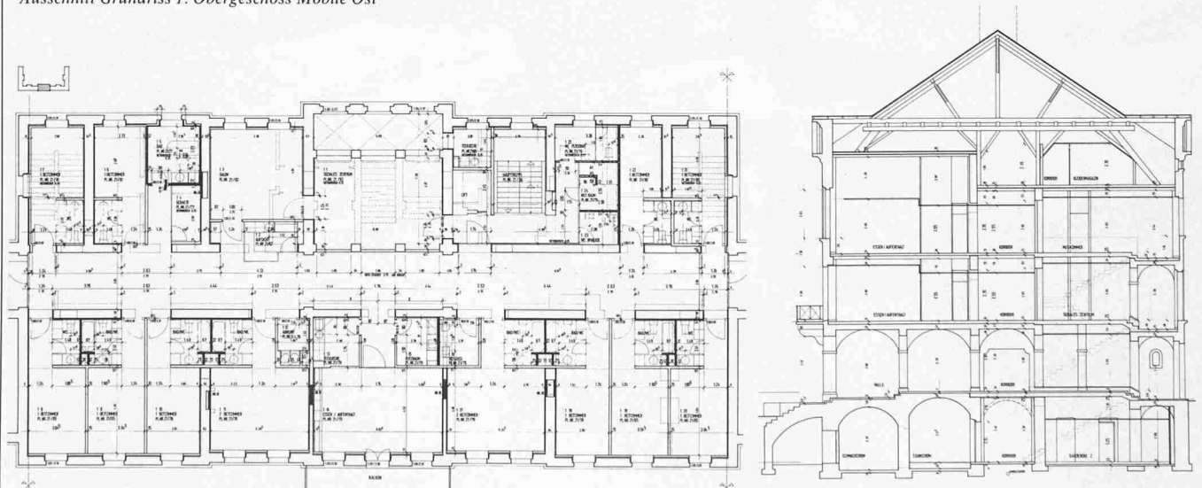
Ausschnitt Grundriss 1. Obergeschoss Mittelbau Privat
