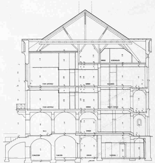
Schnitt durch den Mittelbau
