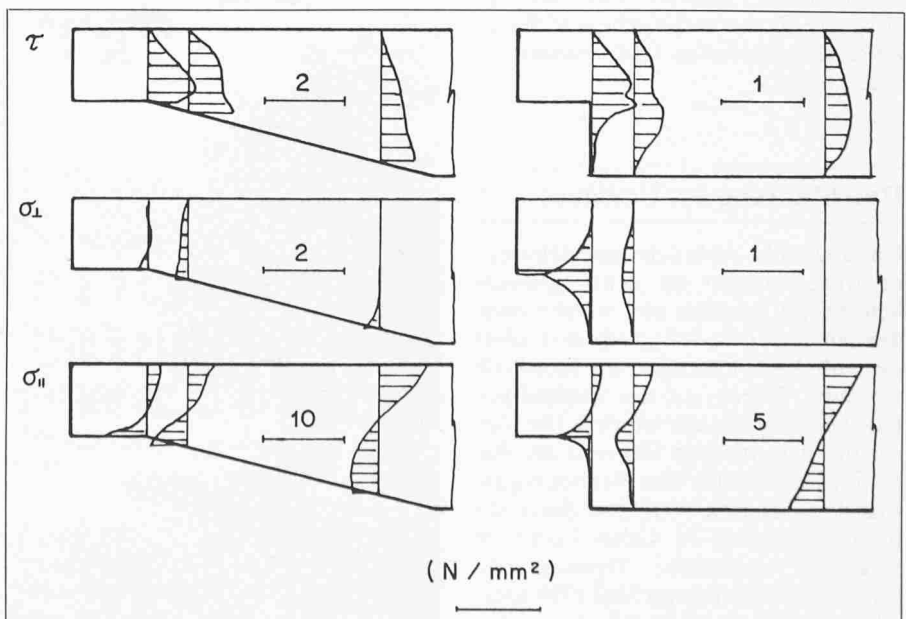
Bild 2. Spannungsverteilung bei Ausklinkung nach [4]
