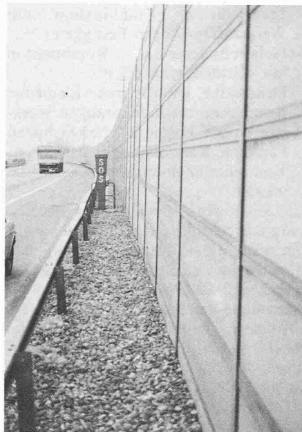
Bild 6. Hohe wetterexponierte Schallschutzwand längs einer Autobahn bei Zürich/ (Schweiz). Die mit mineralischen Pigmenten grün eingefärbten «Duri- panel»-Platten werden durch verzinkte Stahlprofile gehalten
