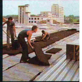
Atmungs-fähige Flachdachisolation
