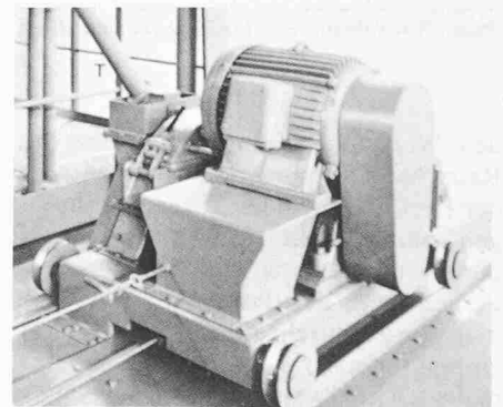
Bild 27. Auf dem Dach des Maschinengehäuses der Anlage zum Peenen von Zahnkränzen mittlerer Grösse hin- und herfahrende Schleuderrad-Einheit: Strahlmittel-Zuführung mittels Teleskoprohr T Photo: Graber und Wenig AG., Neftenbach
