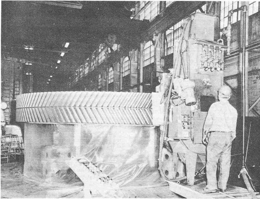
Bild 30. Shot-peenen eines grossen Zahnades von 7100 mm Durchmesser. Auswärtsarbeit. Nach dem Druckluftsystem arbeitende, als semi-portable bezeichnete Spezialausrüstung. Sie ist mit vier in der Strahlkabine eingebauten, eine vertikale Hin- und Herbewegung ausführenden Injektor-Strahlpistolen ausgerüstet, währenddem die Strahlmittelzufuhr mittels Becherwerk nach dem Gravitationssystem erfolgt. Zusätzliche Abdichtungen: Plastiktücher.
