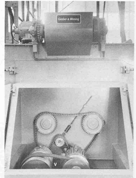
Bild 26. Mit einer auf dem Dach der Maschine aufgebauten, hin- und herfahrenden Schleuderradeinheit ausgerüstete Anlage zum Peenen von Getriebezahnkränzen mittlerer Grösse. Blick in die an der Stirnseite des Werkstückwagens angebaute Antriebsstation für die Drehbewegung der beiden mit einer dicken Gummischicht überzogenen Tragwalzen und des auf ihnen ruhenden zu peenenden Zahnkränzes. Im Vordergrund der Variator V für die Drehzahlregulierung. Darüber ist der auf dem Maschinendach aufgebauten Antrieb für die Fahrbewegung der Schleuderrad-Einheit zu sehen. P: Spannvorrichtung für Kettenantrieb der Drehwalzen Photo: Graber und Wenig AG., Neftenbach
