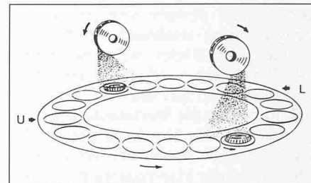
Bild 17B. Prinzipschema eines grossen Satelliten-drehtisches für das Peenen von PKW-Getriebeteilen und Zahnradern, ausgerüstet mit zwei Schleuderrädern von je 25 PS Leistung sowie mit insgesamt 18 Satellitendrehtischen.
