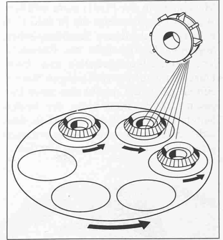
Bild 16 A Die Behandlung von Kegelrädern nach dem Shot-peening-Verfahren auf mit Satellitendrehstischen ausgerüsteten Schleuderradmaschinen
