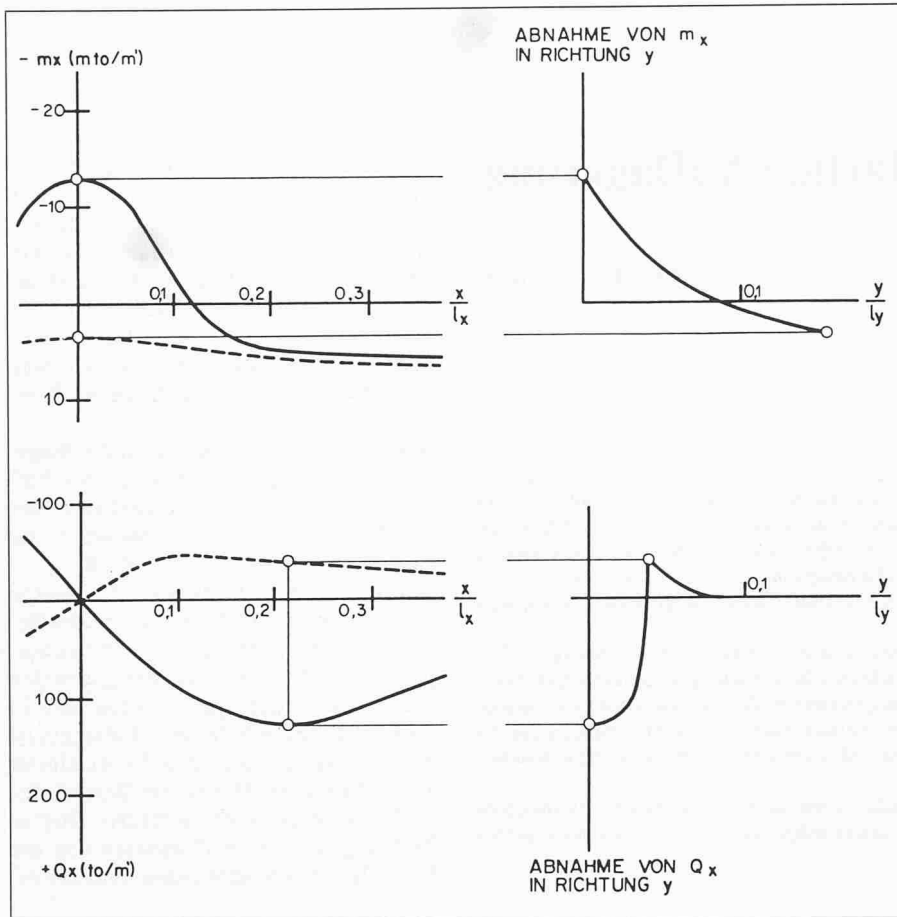
Bild 2. Schnittkraftverlauf in x-Richtung
