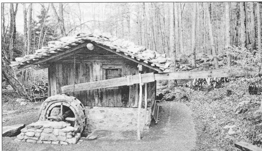
Wassergetriebene Leinsamenstampfe aus Curaglia (GR). In der Kammer befinden sich Gegenstände des ländlichen Gewerbes
