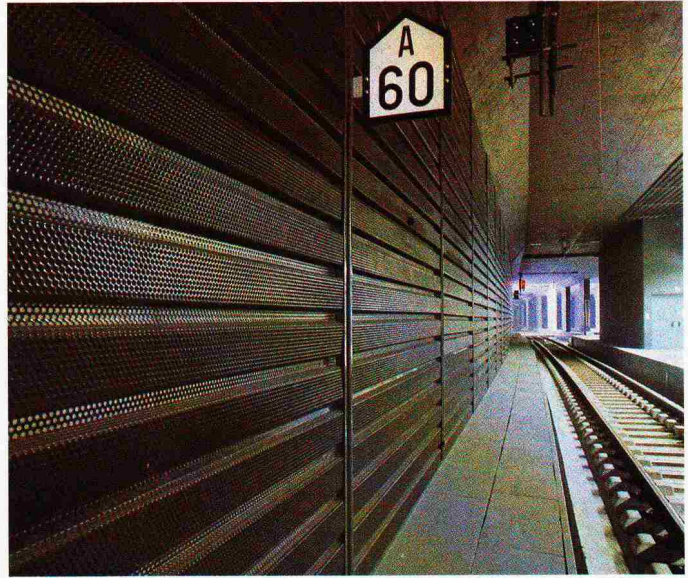
Bild 10. Schallschutzwand im Bereich des Gepäckkaulades
