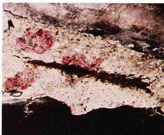
Brücke C. Die Resthaftung (rote Zone) dieser abgedrückten Betonüberdeckung war die Ursache, dass dieser Zustand bis zum Tage der Untersuchung unbekannt blieb
