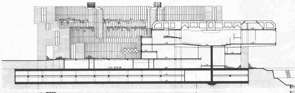
Schnitt B-B 1:1100
