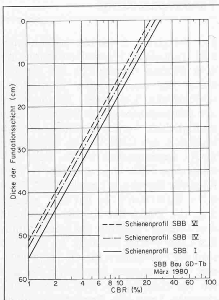
Bild 4. Dicke der Fundamentalschicht in Hauptgleisen unter Holzschwellen
