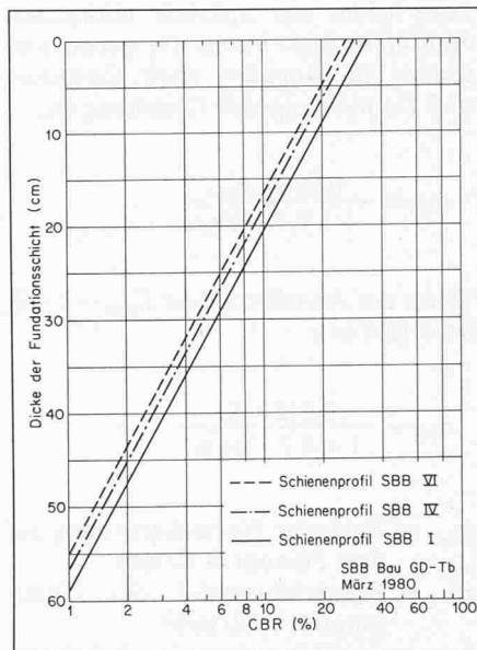
Bild 5. Dicke der Fundamentalschicht in Hauptgleisen unter Zweiblockbetonschwellen
