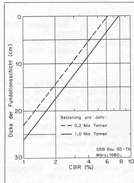
Bild 7. Dicke der Fundamentalschicht in Neben- und Verbindungsgleisen unter Holz- und Stahlschwellen mit Schienenprofil SBB I
