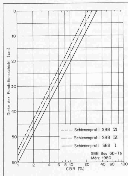
Bild 6. Dicke der Fundamentalschicht in Hauptgleisen unter Einblockbetonschwellen
