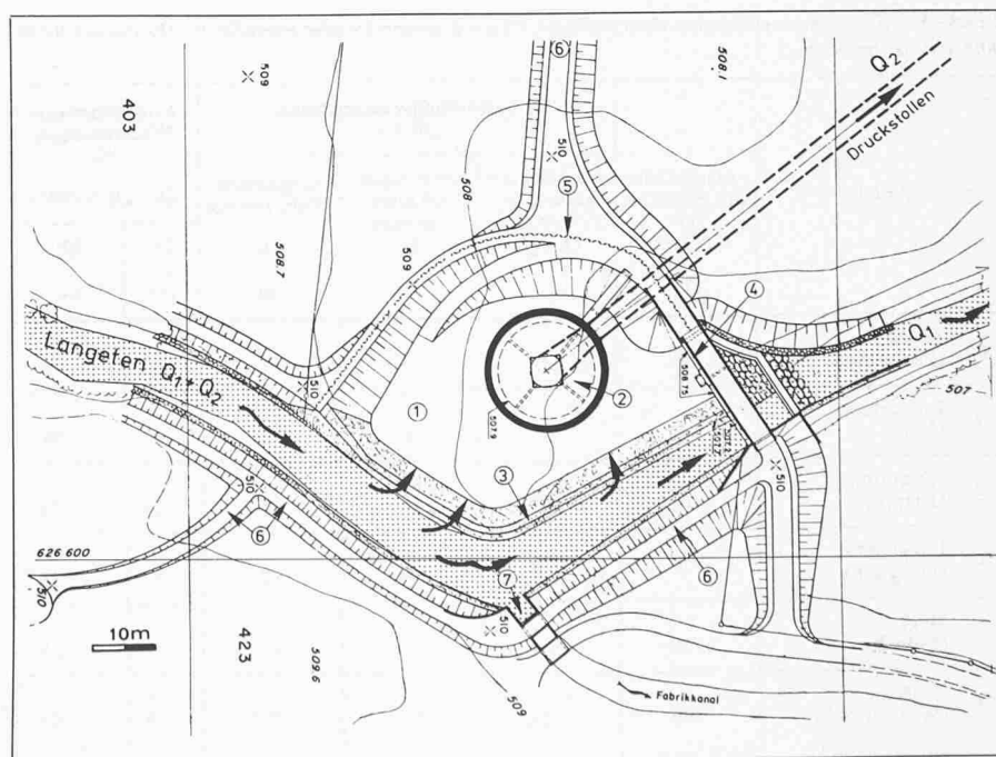
Bild 5. Verzweigungsbauwerk mit Trichterüberfall. Bei einem grösseren Zufluss als 12 \text{ m}^3/\text{s} fällt ein Teil des Wassers der Langeten ( Q_2 ) über das seitliche Streichwehr und staut sich im – den Trichter umgebenden – Becken auf, bis es über die Überfallkante in den Stollen eingeleitet werden kann.
