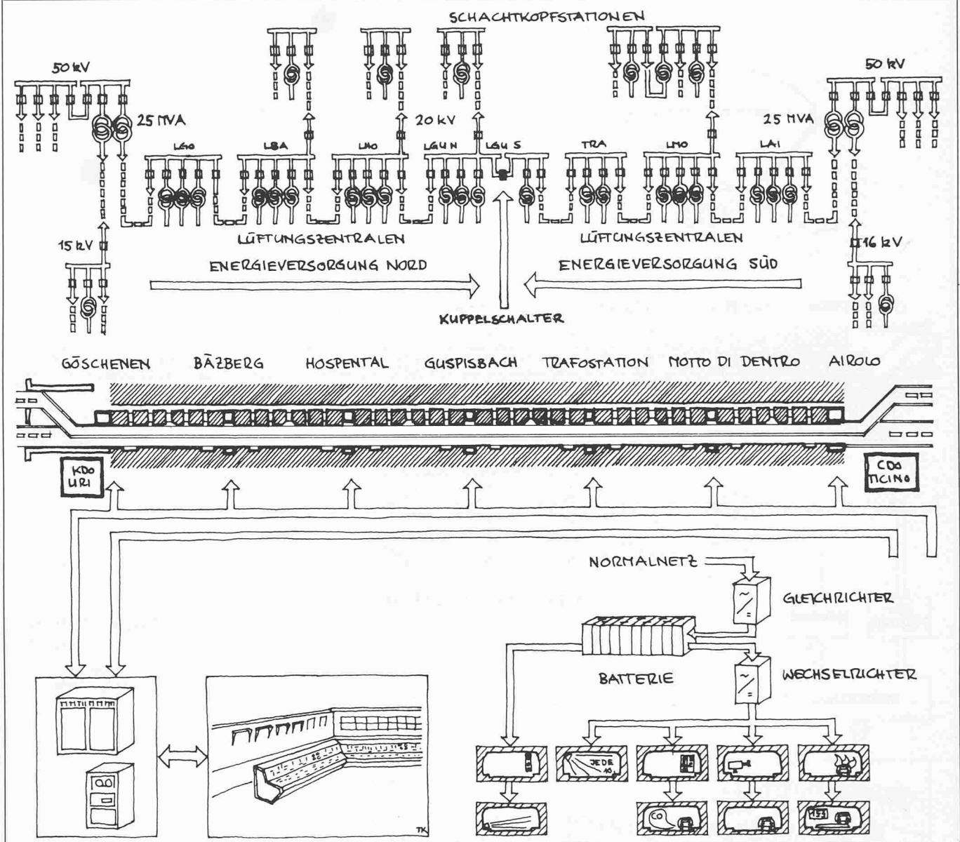
Bild 28. Energieversorgung (schematisch) Figura 28 Alimentazione d'energia (schematica)
