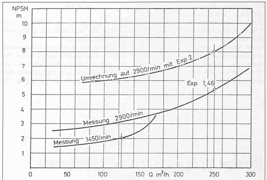
Bild 10. NPSH-Versuchswerte bei 1450 und 2900/min Den ausgezogenen Versuchswerten, die für Q_{\text{opt}} einen Umrechnungsexponenten 1,46 ergeben, sind strichpunktiert die theoretischen Werte mit Exponent 2 gegenübergestellt
