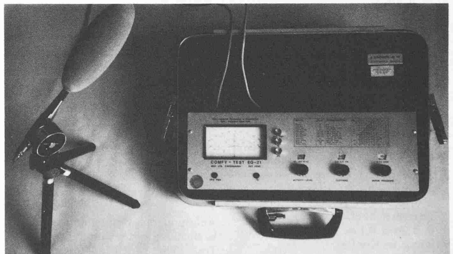
Bild 1. «Comfy-Test»-Gerät EQ-21. Links Modellkörper, der die Haut des Menschen simuliert; rechts elektronischer Messeil
