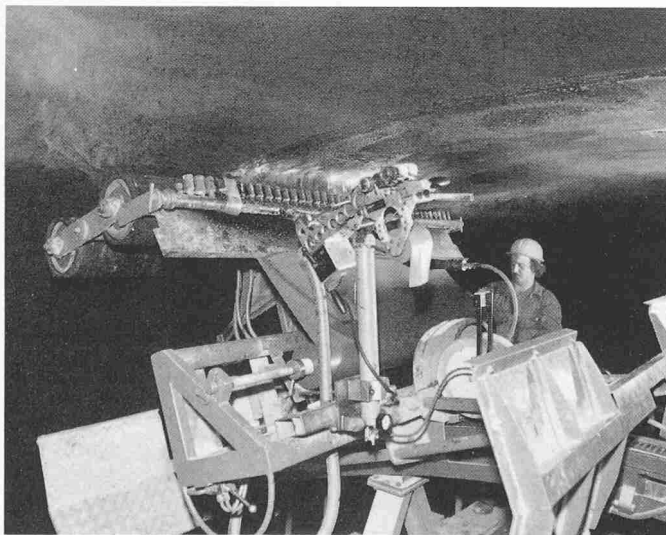
Bild 3. Los West: Aufkleben der Gewölbeisolation auf das Tübbingaussengewölbe
