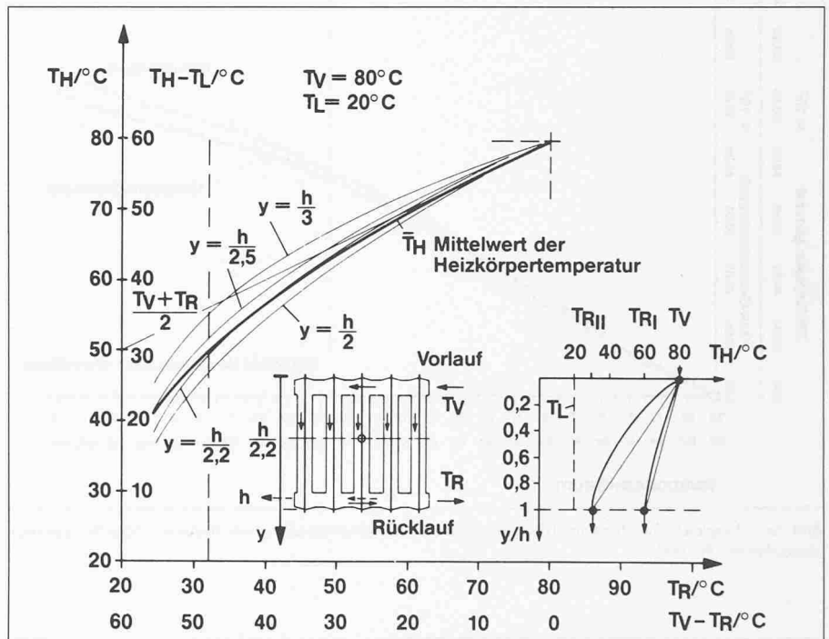
Bild 6. Heizkörpertemperatur als Funktion der Temperatururspreizung zwischen Vor- und Rücklauf
