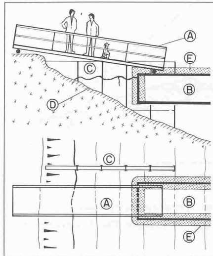
Bild 7. Abschlüsselemente für Schwimmhäfen, A Rollbrücke, B Schwimmelemente, C Abschlusswand, D Seegrund, E Bewegungsbereich der Mole
