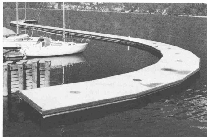
Bild 4. Hafenanlage Gäsi am Walensee, Ausbildung als Schwimmole
