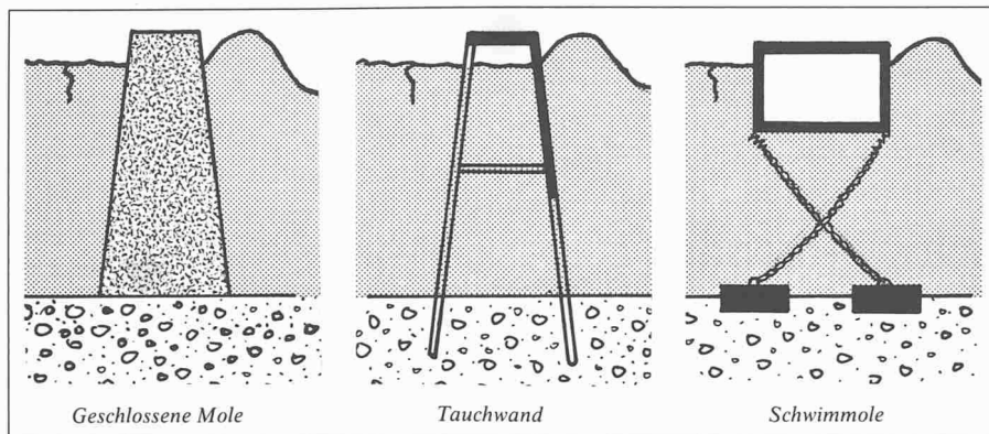
Bild 1. Drei für Hafenbauten in der Schweiz oft verwendete Molentypen
