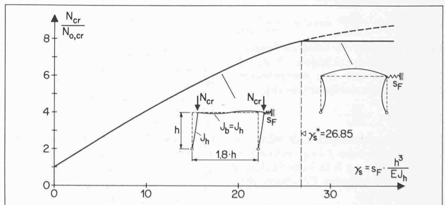
Bild 2. Verlauf der Verzweigungslast N_{cr} des querverfederten Rahmens in Funktion des Steifigkeitswertes \gamma_s ; Definition der Mindeststeifigkeit \gamma_s^*
