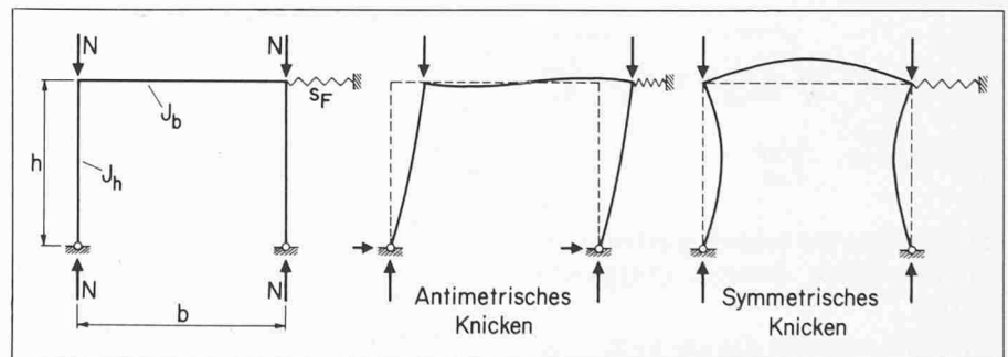
Bild 1. Knickformen beim querverfederten Rahmen
