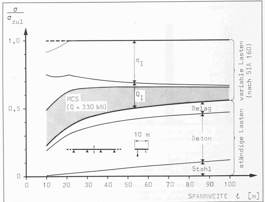
Bild 3. Anteile der Spannungen von Verbundbrücken bezüglich der Grenzlaster nach SIA 160 in Funktion der Spannweite. Punktierte Fläche entspricht einer zweiachsigen Modelllast MCS nach Bild 6
