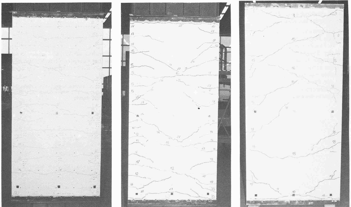
Bild 8. Rissentwicklung
