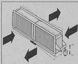
Q-dot-Wärmetauscher können durch eine einfache Kippeinrichtung leistungsregelt werden, zum Beispiel von Heiz- auf Kühlbetrieb oder konstante Ausblastemperatur
