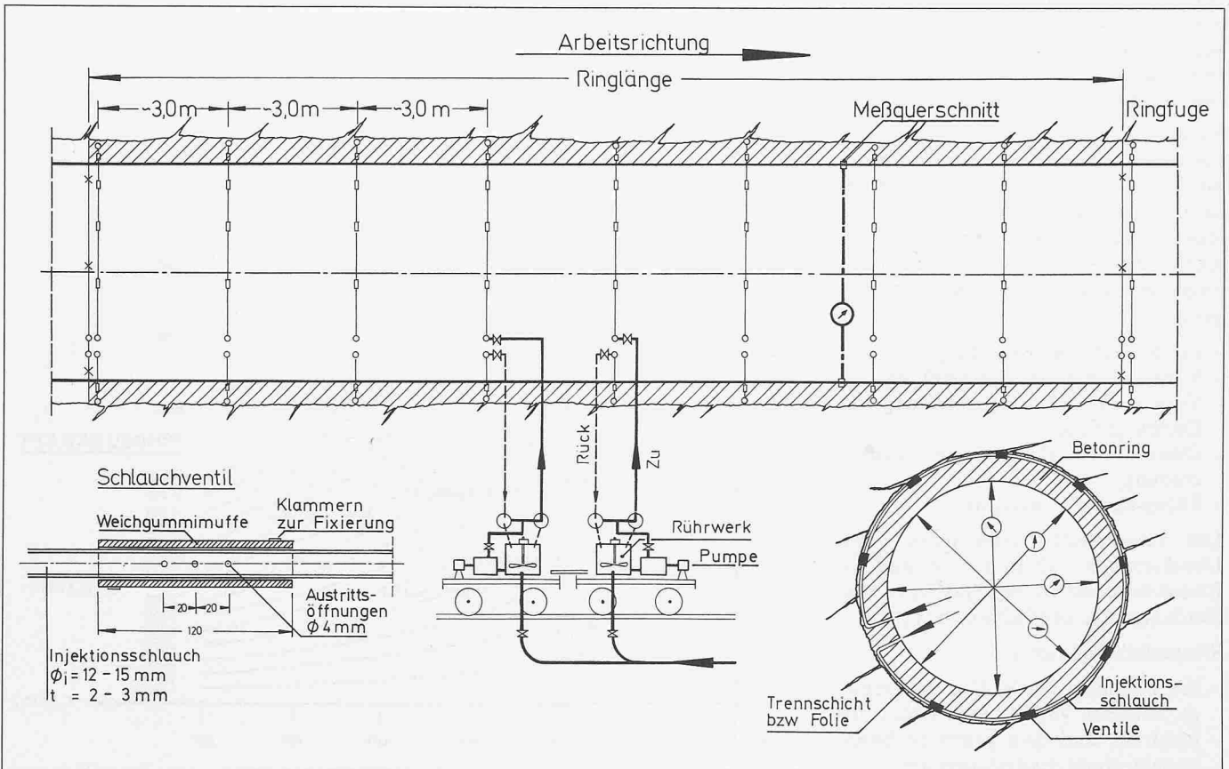
Bild 3. Das Tiwag-Spaltinjektionsverfahren
