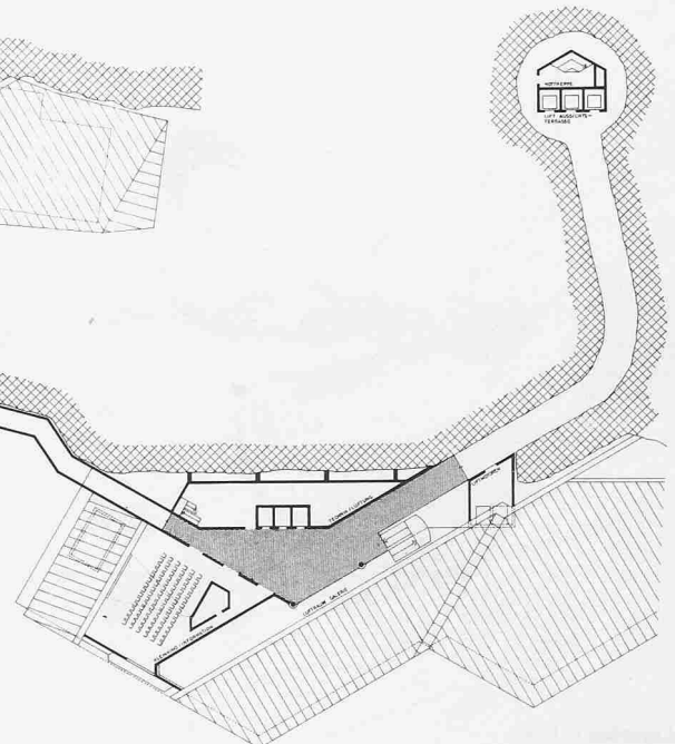
Niveau 3470.00, Zugang Aussichtsterrasse
