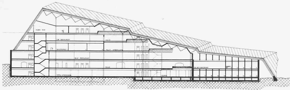
Längsschnitt Berghaus
