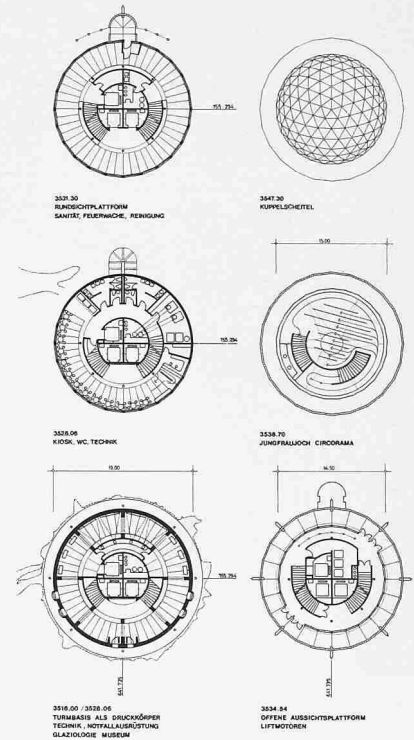
Grundriss Aussichtsterrasse 1:1000
