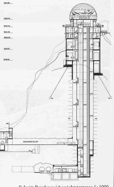
Schnitt Berghaus/Aussichtsterrasse 1:1000
