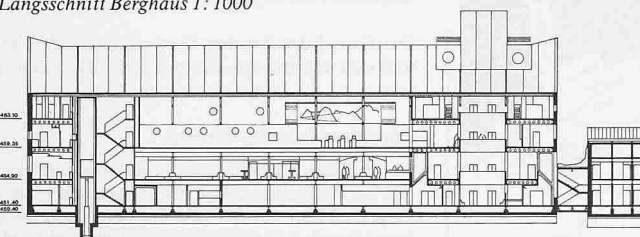
Längsschnitt Berghaus 1:1000
