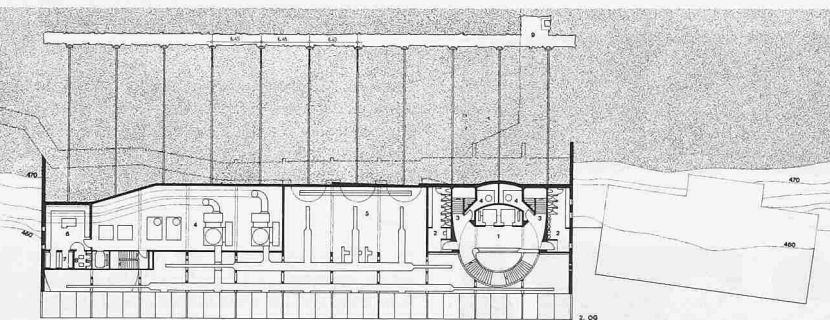
Längsschnitt Berghaus 1:1000
