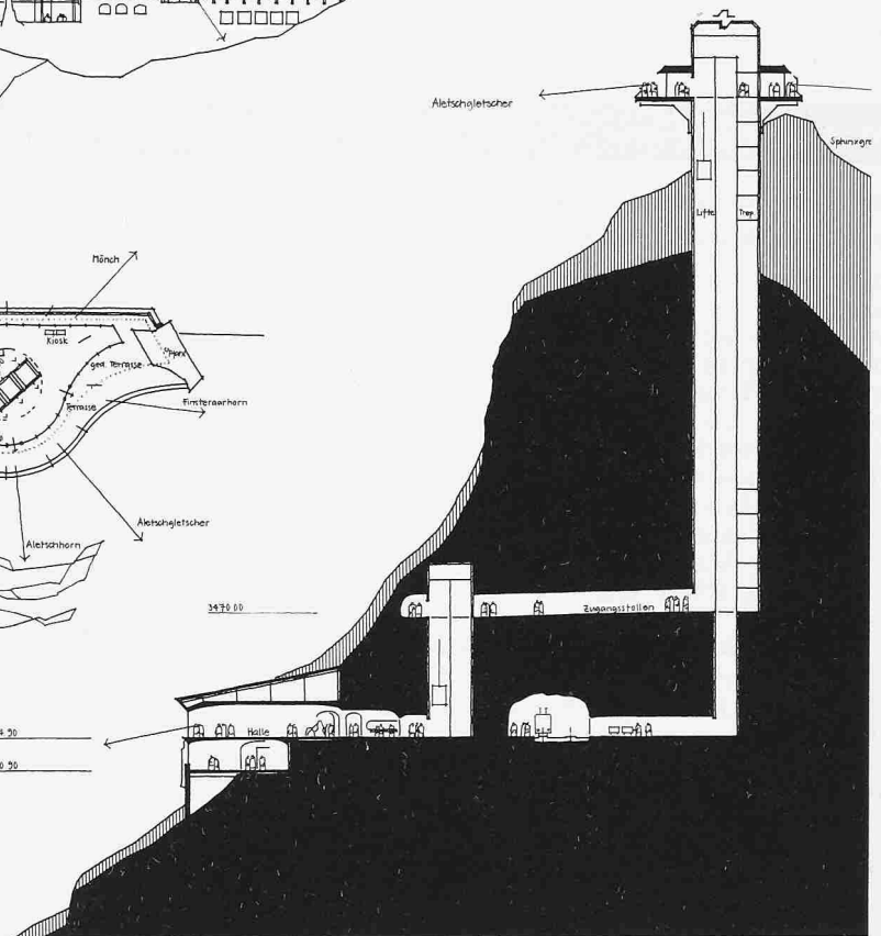
Schnitt Berghaus/Aussichtsterrasse 1: 1000
