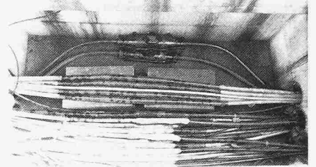
Bild 8. Spleisschacht, geöffnet
