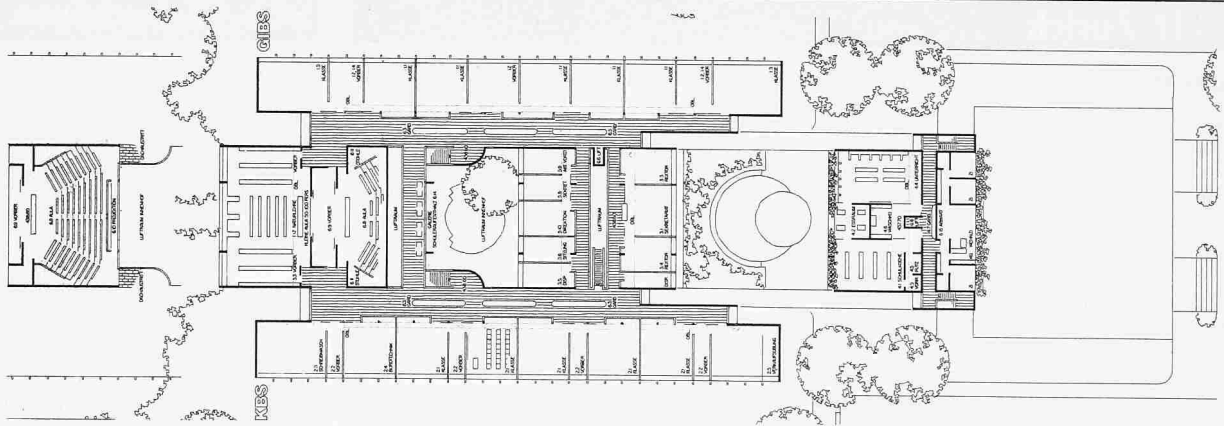
Grundriss Obergeschoss 1: 1100
