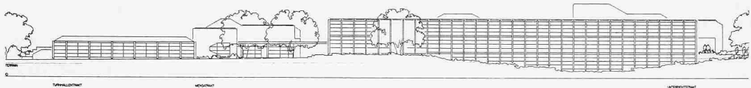
Ansicht von Osten 1: 1100
