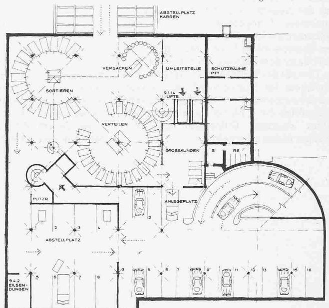
Grundriss 1. Untergeschoss 1:600
