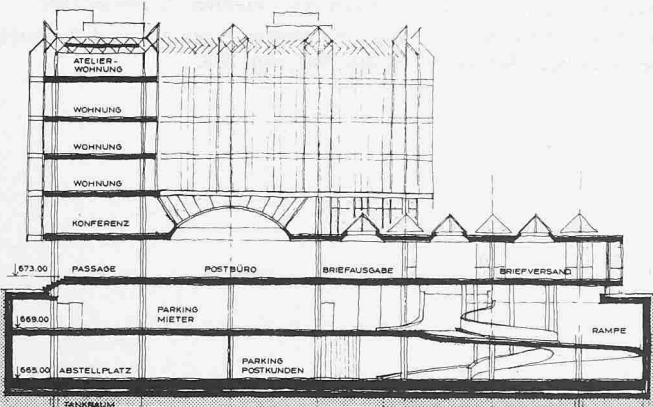
Schnitt 1:600
