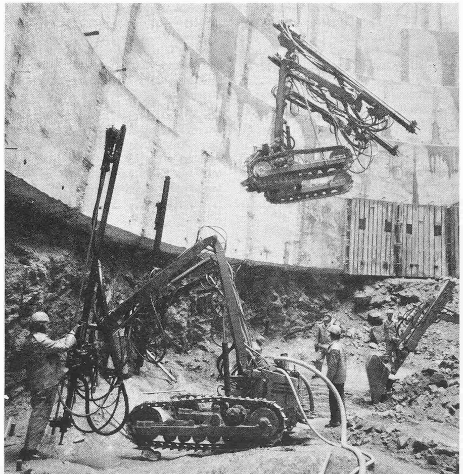
Bild 10. Abteufen des 82 m tiefen Schachtes für das Kraftwerk Kühtai; Felswand unter der Betonauskleidung 3,00 m hoch freistehend
