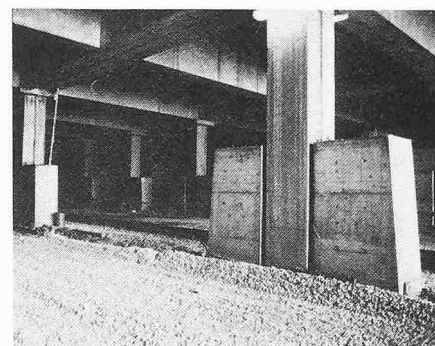
Bild 6. Durch Anprallböcke geschützte Stützen Überbauung im Weichenbereich des Franz-Josef-Bahnhofs (vgl. auch Tabelle 1)
