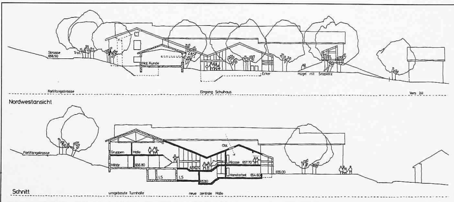
Ansichten, Schnitte 1:900
