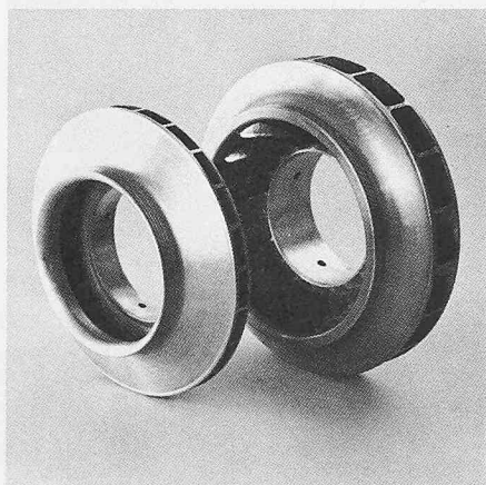
Kompressorlaufräder (radial)
