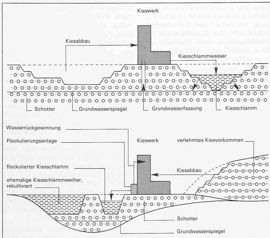
Bild 2. Prinzipschema einer Kiesgewinnung. Oben: Schottervorkommen Unten: Verlehmt Kiesvorkommen
