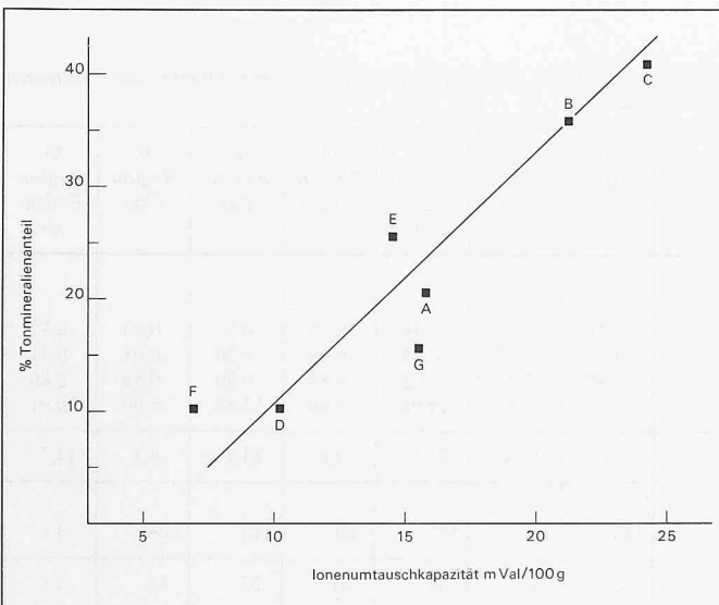
Bild 5. Zusammenhang zwischen Ionenaustauschkapazität und Tonmineralgehalt der Korngrössenfraction <0,063 mm
