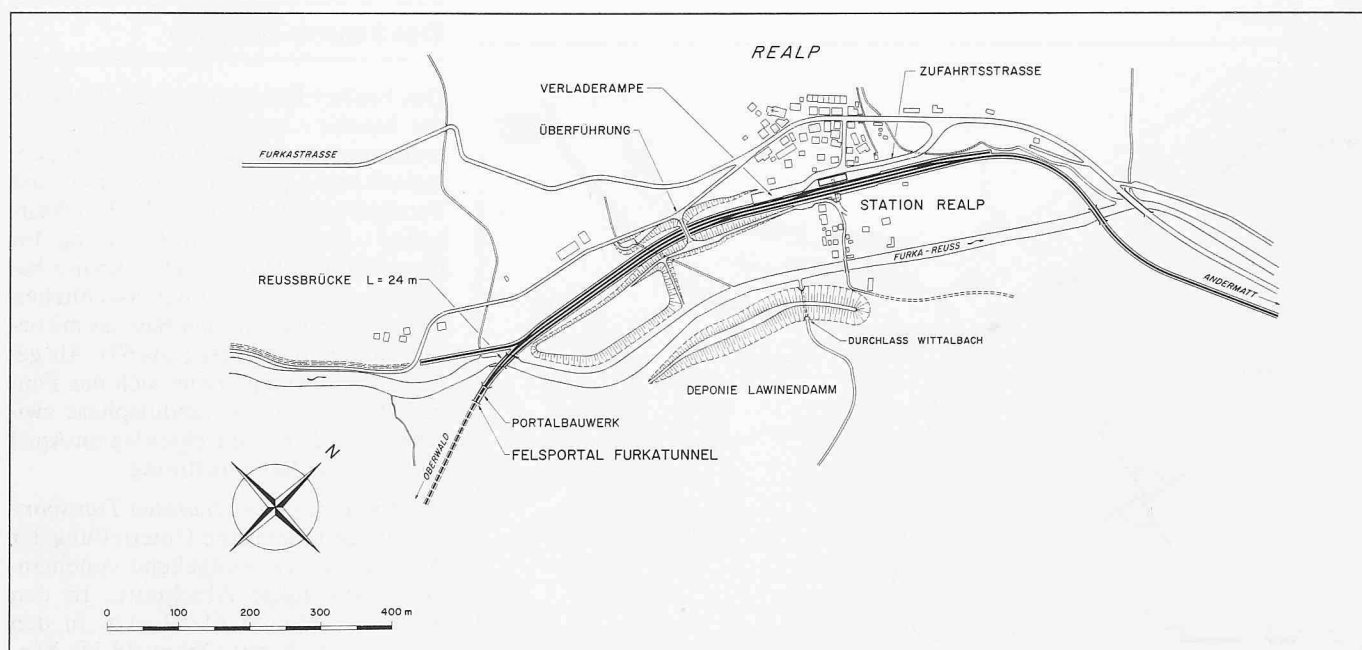
Bild 3. Situation Zufahrt Realp
