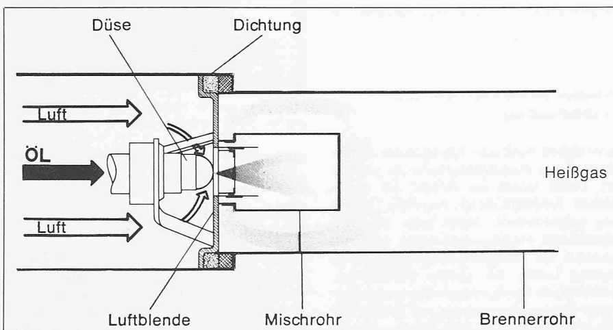
Schnitt durch MAN-Ölbrenner mit totaler Verbrennung, hoher Energieausbeute und niedrigem Schadstoffanteil
