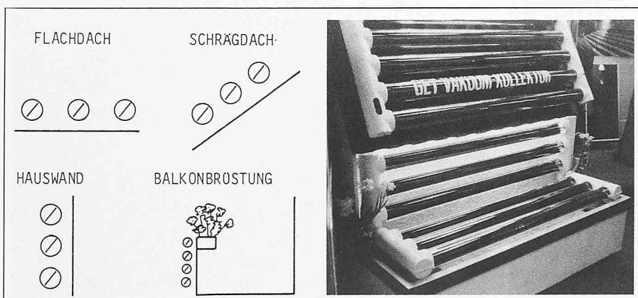
Vakuum-Sonnenkollektoren
