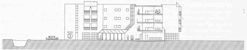
Schnitt A-A, 1:600
