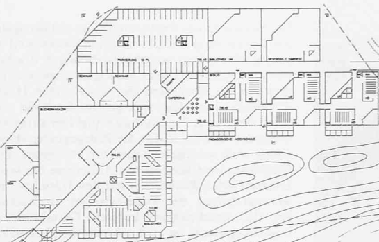
Geschoss B 1: 2500
