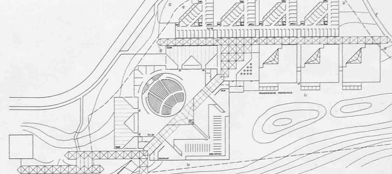
Geschoss D 1: 2500
