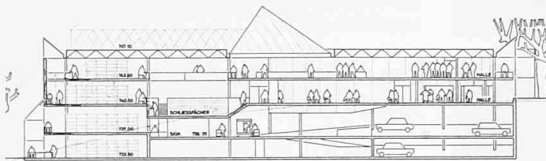
Schnitt B-B 1: 900
