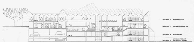
Schnitt C-C 1:900
