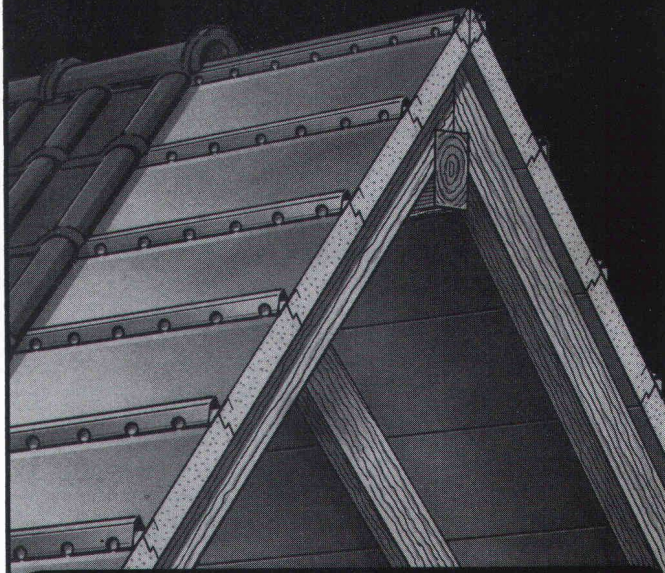
Modell Riffelblech
