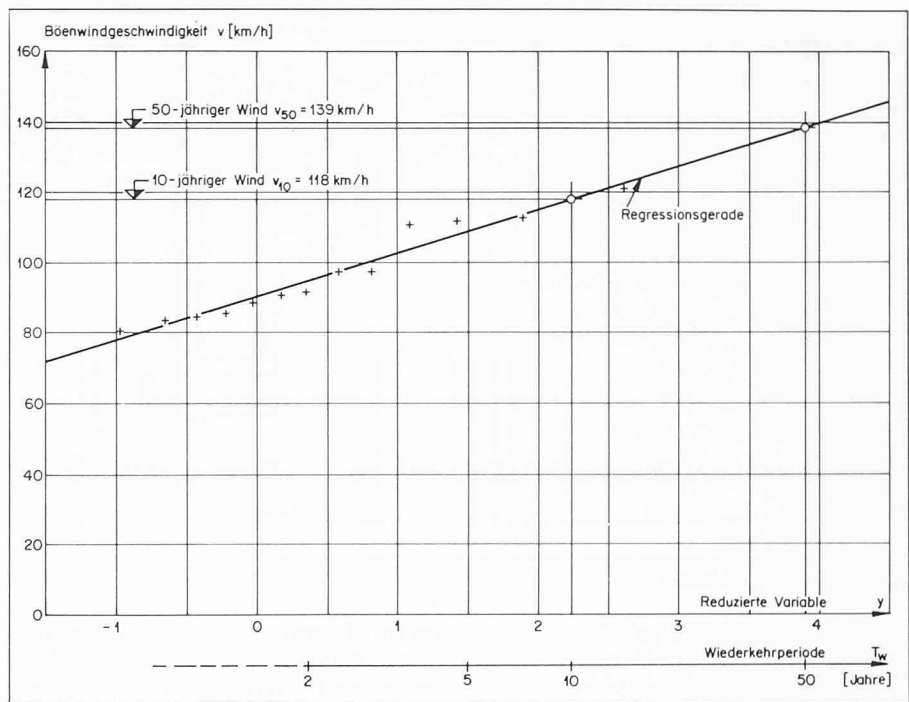
Bild 6. Windgeschwindigkeitsextrapolation für Lugano (Grundlage: 13 Jahresmaxima)
