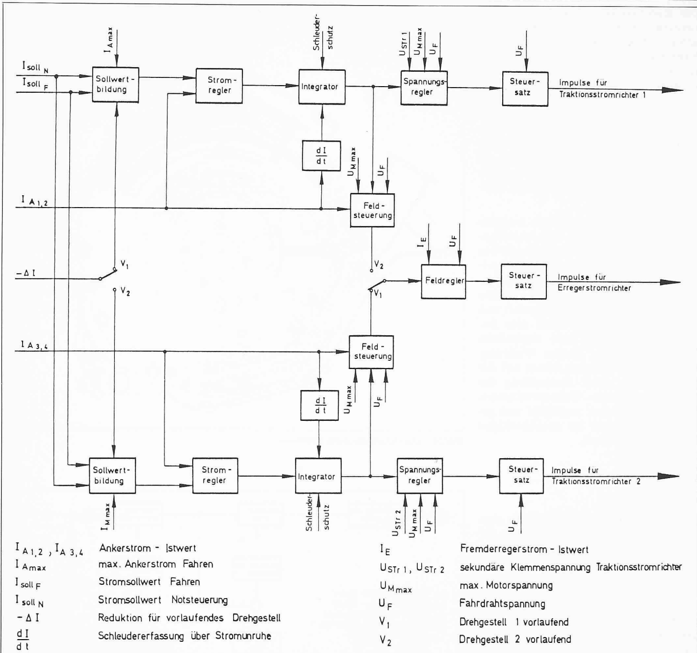
Bild 26. Blockscheema Antriebssteuerung für Fahren. Schalter in Stellung entsprechend «Vorwärts 1» gezeichnet
