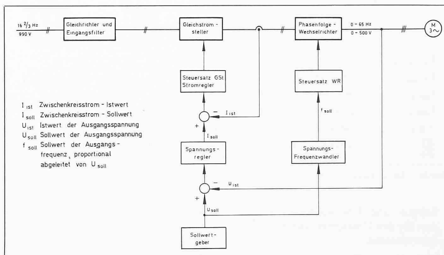
Bild 25. Hilfsbetriebeumrichter. Blockscheema
