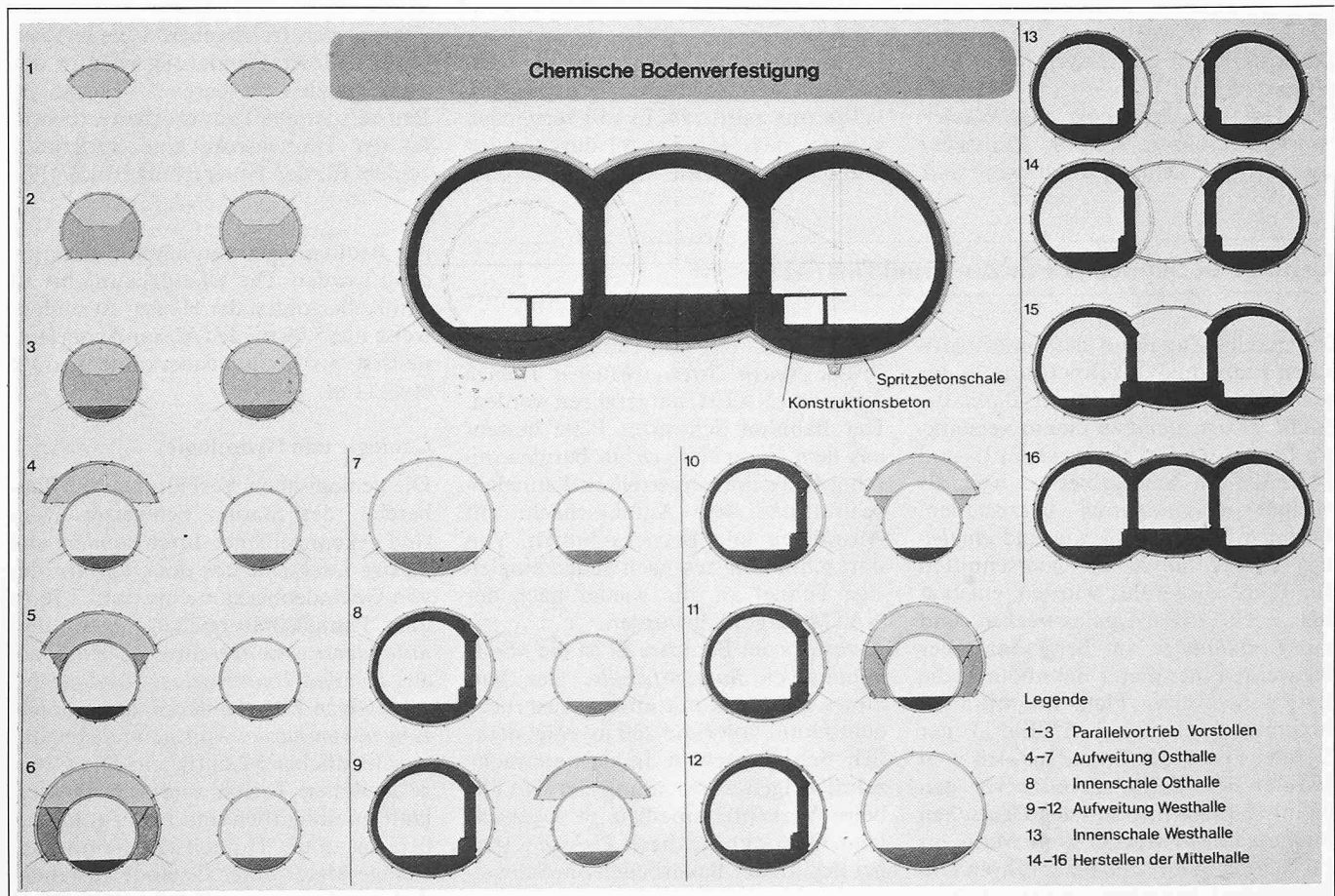
Bild 2. Arbeitsablauf bei Bau des U-Bahn station Schweizer Platz mit insgesamt über 230 m 2 Ausbruchquerschnitt
