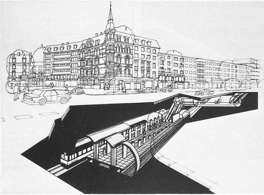
Bild 1. U-Bahn station Schweizer Platz in Frankfurt/Main
