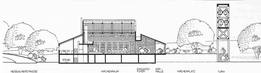
Längsschnitt 1:700
