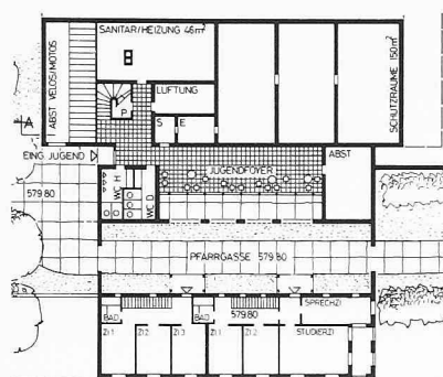
Untergeschoss Kirche/Obergeschoss Pfarrhaus
