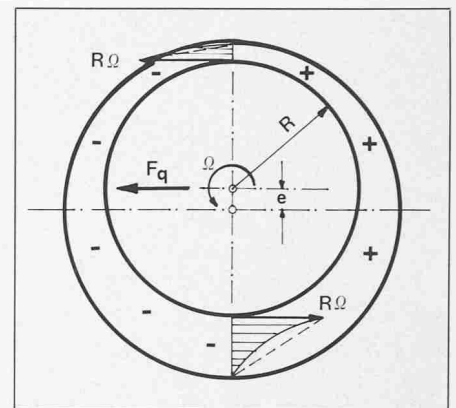
Bild 9. Kraft auf Welle bei festgehaltenem Wellenzentrum
