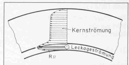
Bild 12. Profil der Umfangsgeschwindigkeit im Labyrinth
