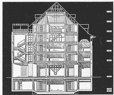
Erdgeschoss, 1. Obergeschoss, Schnitt
