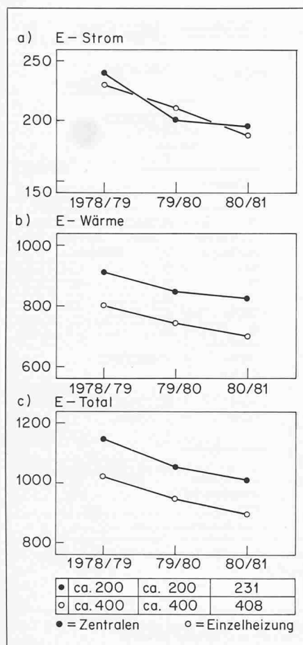
Bild 3. Verbrauchsentwicklung 1978 bis 1981
