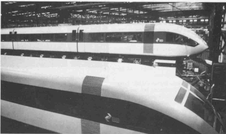
Die Aufnahme zeigt den weitgehend fertiggestellten Transrapid 06 in den Werkhallen von Krauss-Maffei kurz vor der Überführung zur Versuchsanlage im Emsland. Im Auftrag des Bundesministeriums für Forschung und Technologie errichtet das Konsortium Magnetbahn Transrapid zur Erprobung der Magnetschwebetechnik im Dauerbetrieb eine Versuchsanlage im Emsland. Ab Sommer 1983 wird dort der aus zwei Sektionen bestehende, insgesamt 54 m lange, magnetisch getragene und geführte, mit Langstatorantrieb ausgerüstete und für 200 Personen ausgelegte «Transrapid 06» bei Geschwindigkeiten bis zu 400 km/h erprobt werden (Aufnahme: Krauss-Maffei, München).
